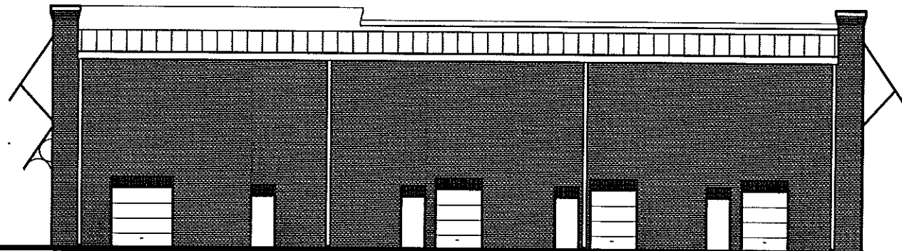
1 A1.0 EAST ELEVATION SCALE: 1/8"=1'-0"
